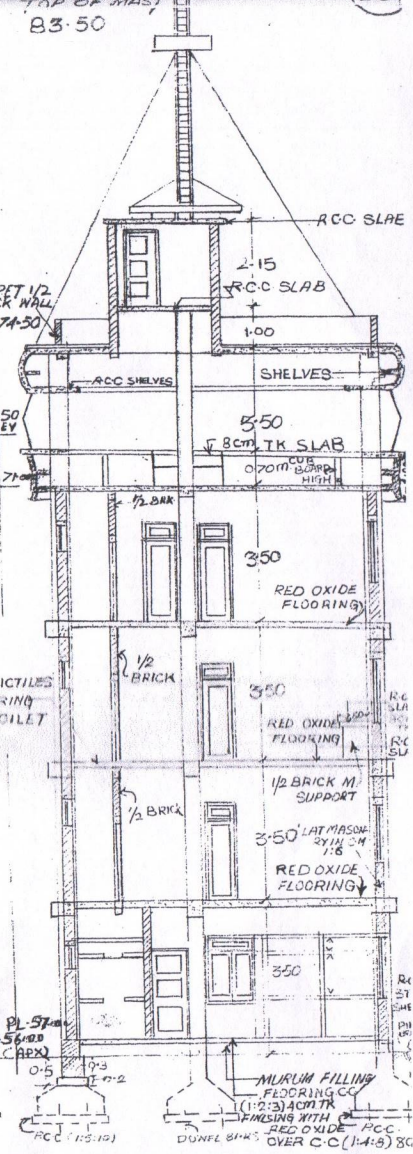
SECTION A-B
